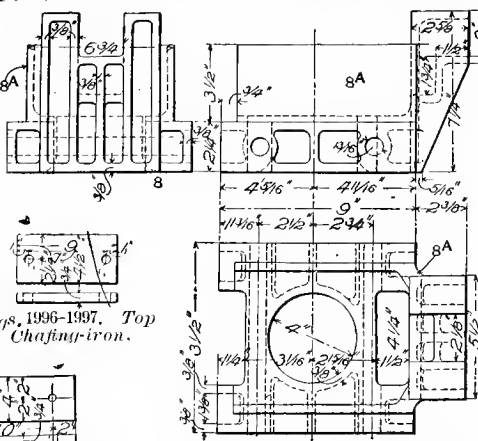
Figs. 1998-1999. Buffer-plank Face-plate.
